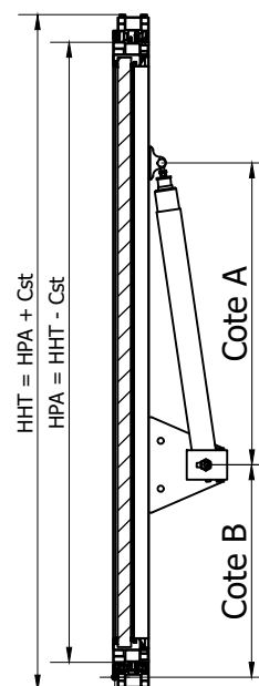
B-B ( 1:10 )
