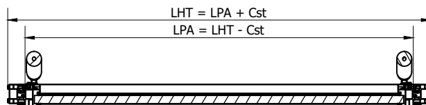
A-A ( 1:10 )
